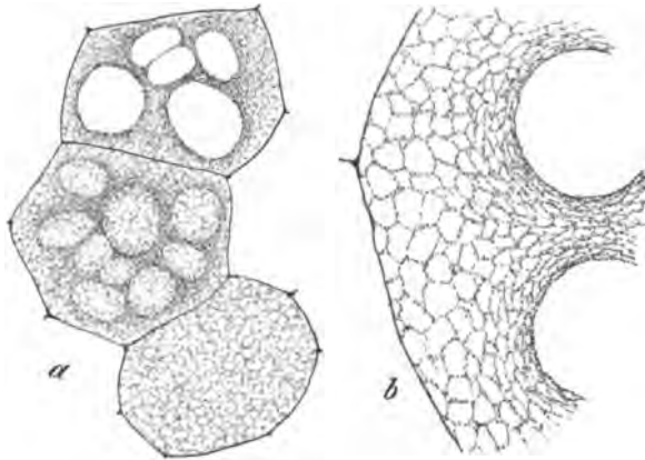
Fig. 20. Secundäre Vacuolisirung von Gerüststrukturen. Casein 2-proc. in 0,2 KOH in Hollunderschnitten mit 0,5-proc. Essigsäure gefällt, wird zuerst schön weitmaschig gerüstig, aber infolge partieller Lösung groblöcherig, vacuolig, die Lamellen zwischen benachbarten Vacuolen und die Umsäumung dieser besteht aus zusammengepressten Gerüsten. a Drei Markzellen, neben einander, die untere das reine Gerüstwerk zeigend, die obere den Durchschnitt durch die groben Lacunen, die mittlere eine Aufsicht, um zu zeigen, dass die Löcher und Lacunen wirklich ringsum von der gerüstigen Caseinfällung umgeben sind. (Vergr. 175.) b Ein Stück bei sehr starker Vergrößerung; die weitmaschigen Gerüste, nicht Schaumstrukturen, aus gefälltem Casein werden an der Peripherie der Lacunen enger, sie sind durch die sich ausdehnenden „Vacuolen“ zusammengepresst, so dass eine Vacuolenhaut entstanden ist. Auch in dem Isthmus zwischen den beiden Lücken ist diese Wirkung deutlich zu sehen. (Vergr. 1500.)
